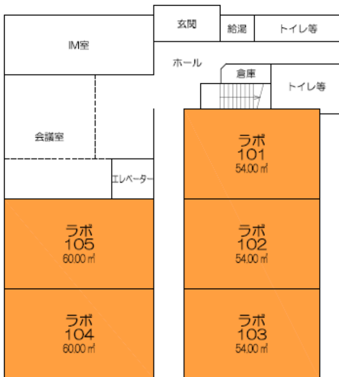
3階平面図
