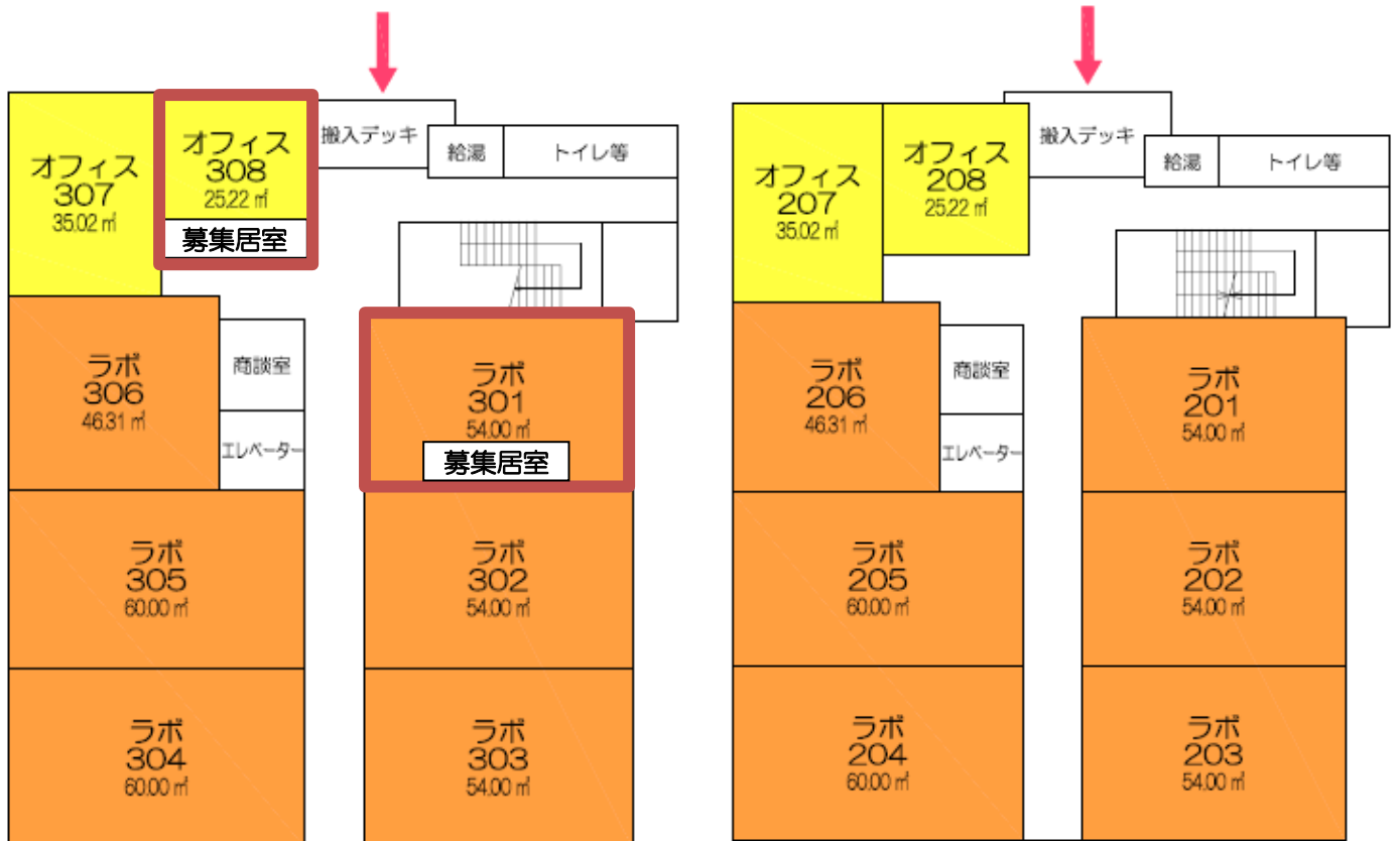
3階平面図
