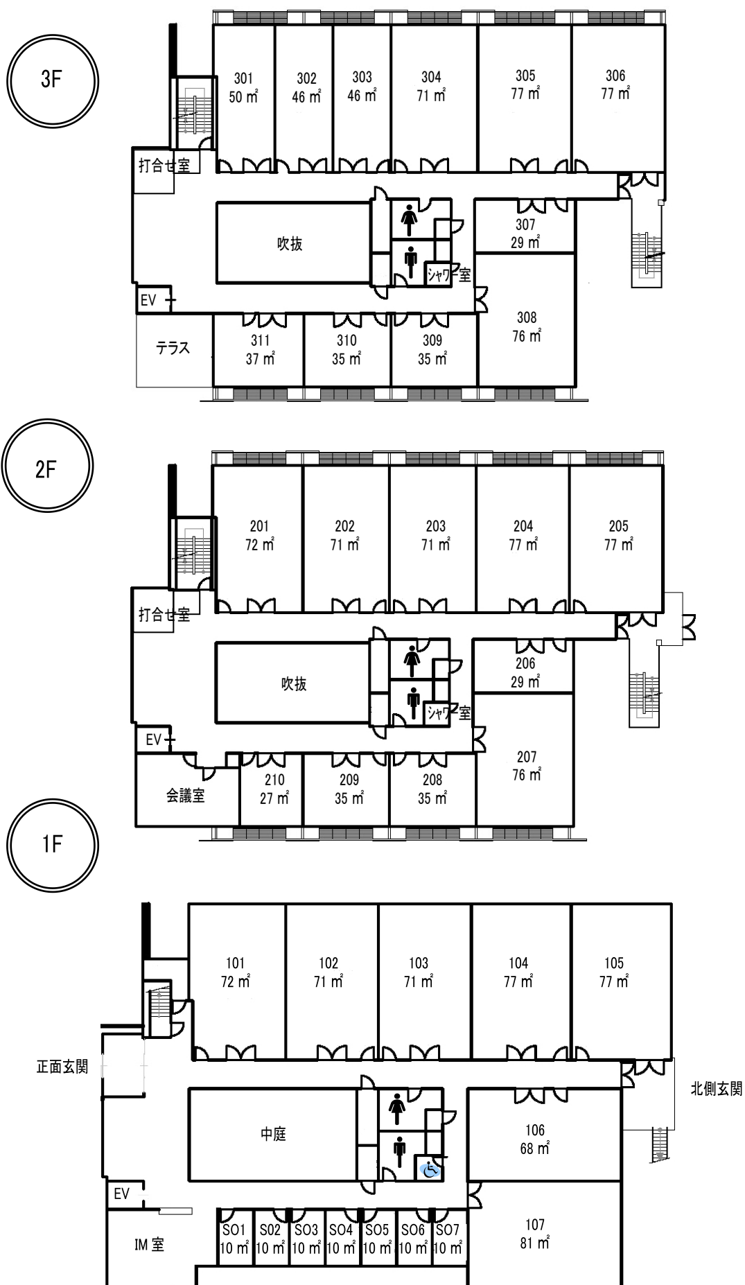
別紙2 京大桂ベンチャープラザ(北館) 間取り図
