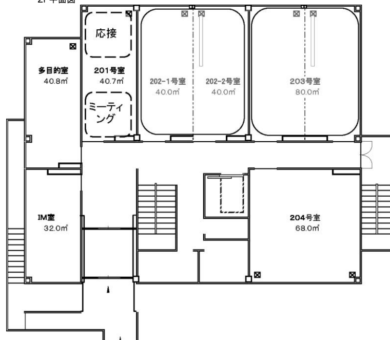
2F平面図
