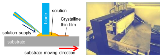
連続エッジキャスト法(左)及び装置(右)
