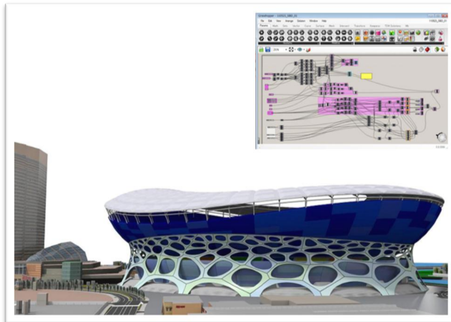
図1:建造物の生体工学的設計のトライアル例
