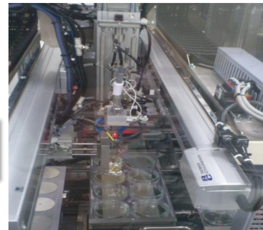
◎細菌自動培養装置
