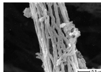
図2 SEM像: 金属が酸化され、鞘の外側に結合している
