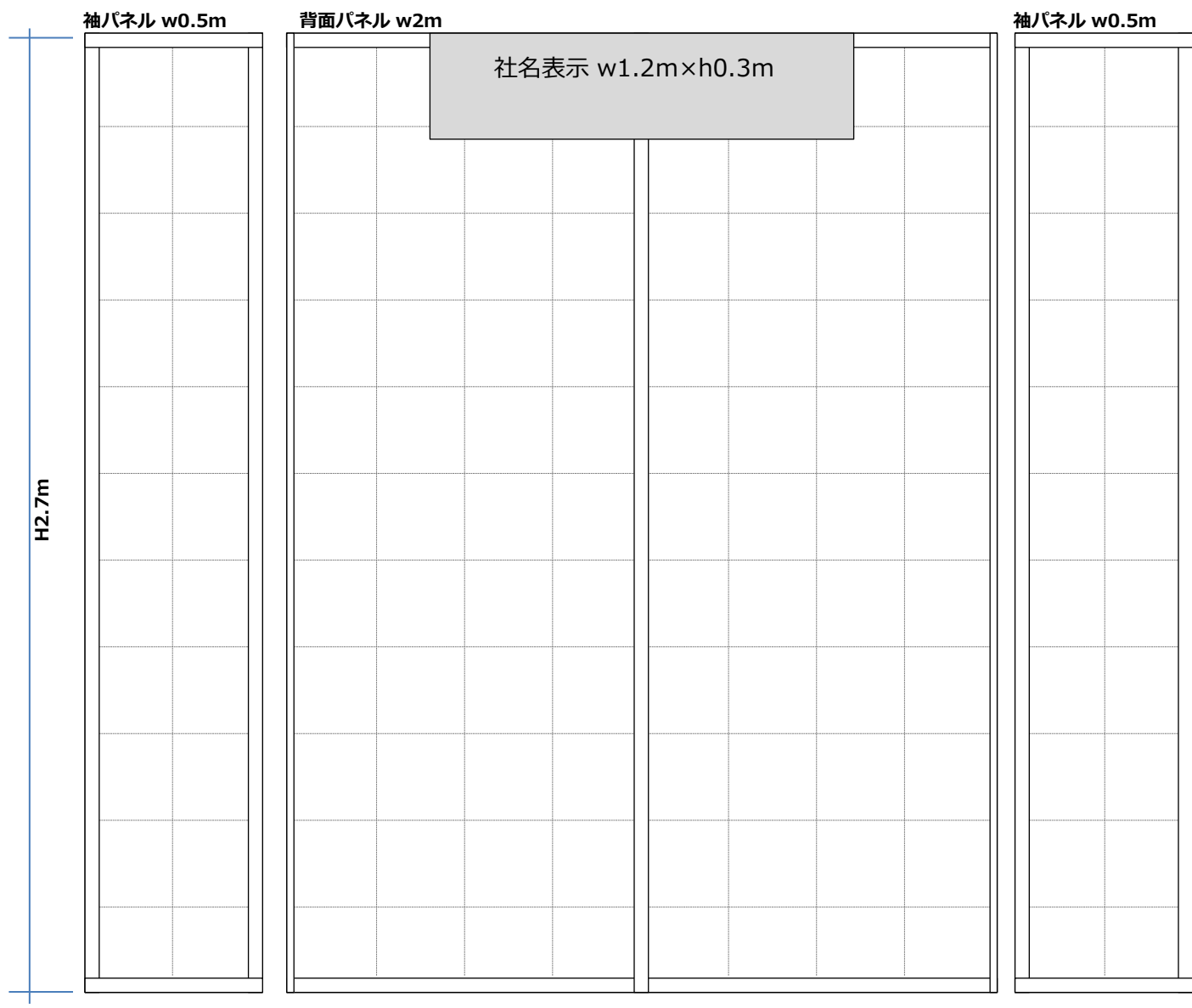
立面図 幅2m×高さ2.7m
