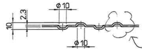
エンボス配置詳細 (S=1:2)
