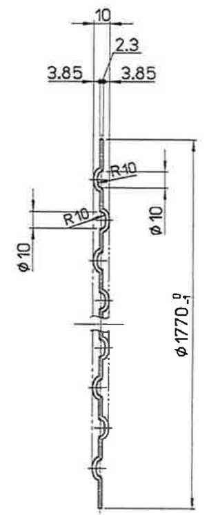
A-A断面 (S=1:2)
