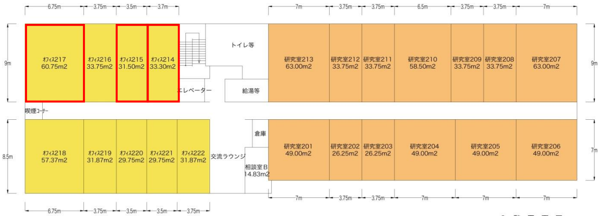
2階平面図
