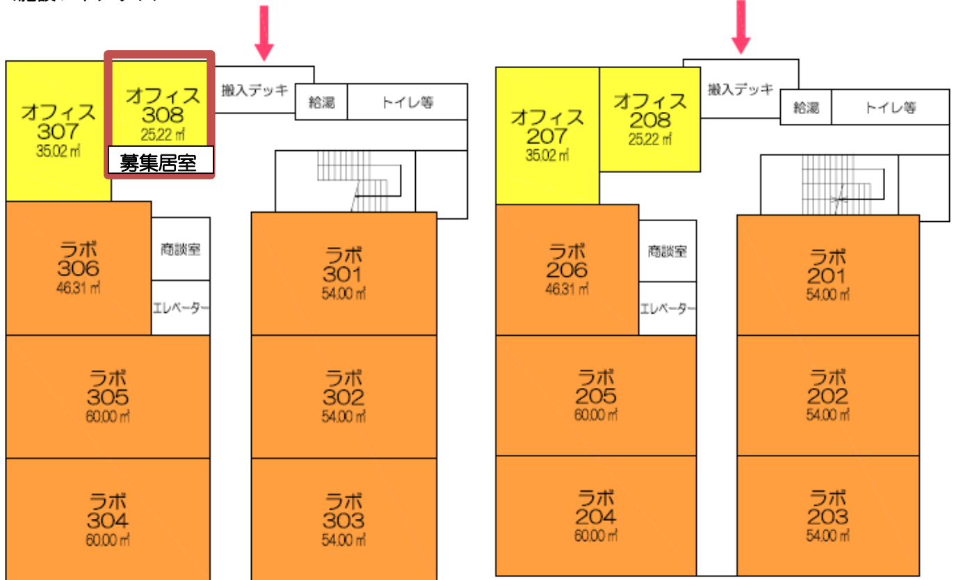
2階平面図
