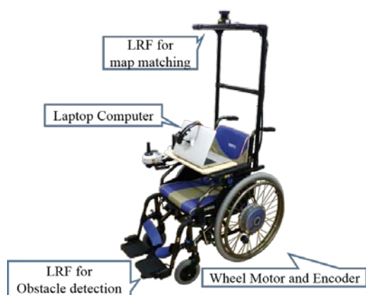
図1 自律走行可能な車椅子
