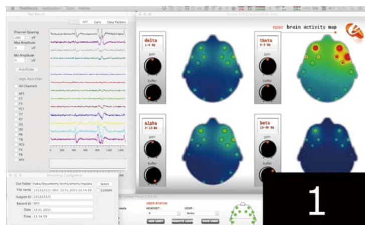
図2 脳波測定ツール
