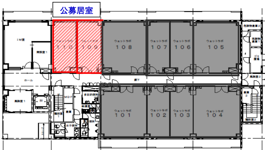
1階平面図
